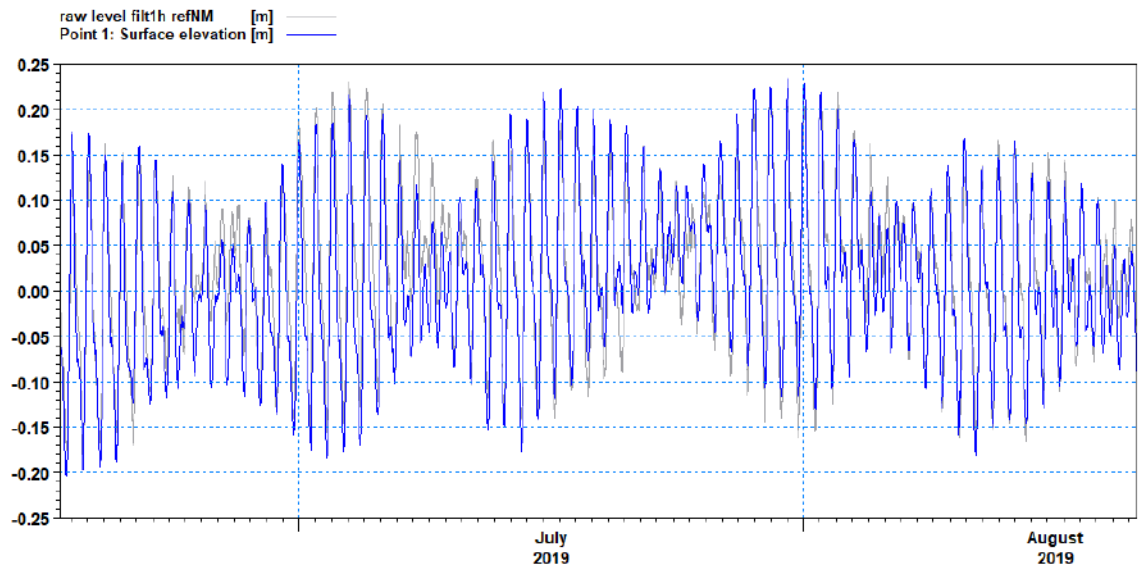
Figure 4.3 Niveaux d'eau (en m par rapport au niveau moyen) modélisés (en bleu) et mesurés au marégraphe de Saint-Martin (en gris) en été 2019 (Réf. /1/).
