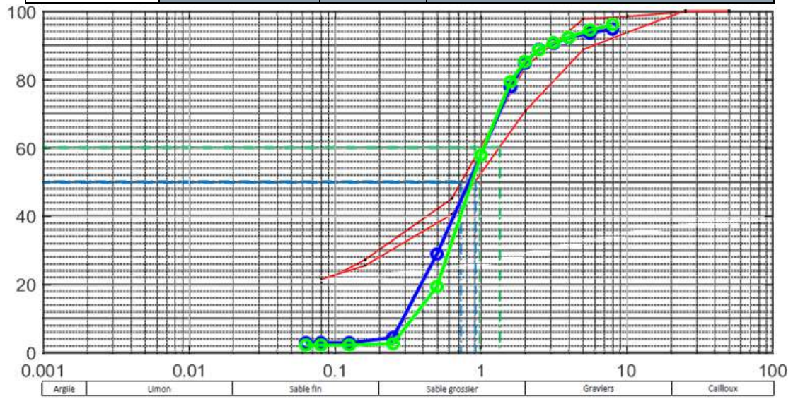
Figure 4.46 Courbes granulométriques des échantillons Ca7 – 0.5 m et Ca7 – 2.5 m (rouge), moyenne de la plage de Sandy Ground (bleu) et de la plage de Galisbay (vert).
