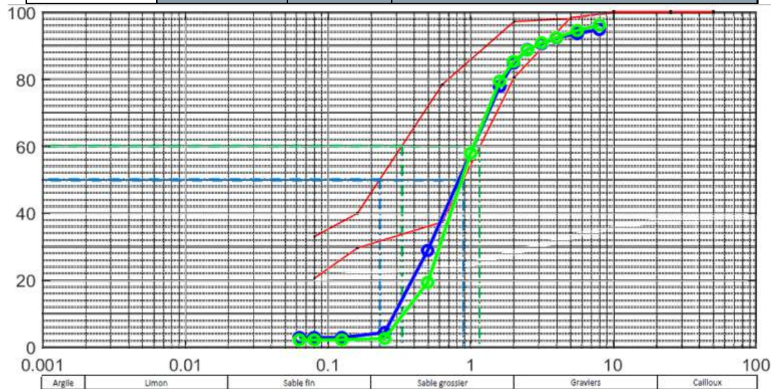
Figure 4.40 Courbes granulométriques des échantillons Ca1 – 1.5 m et Ca1 – 2.5 m (rouge), moyenne de la plage de Sandy Ground (bleu) et de la plage de Galisbay (vert).
