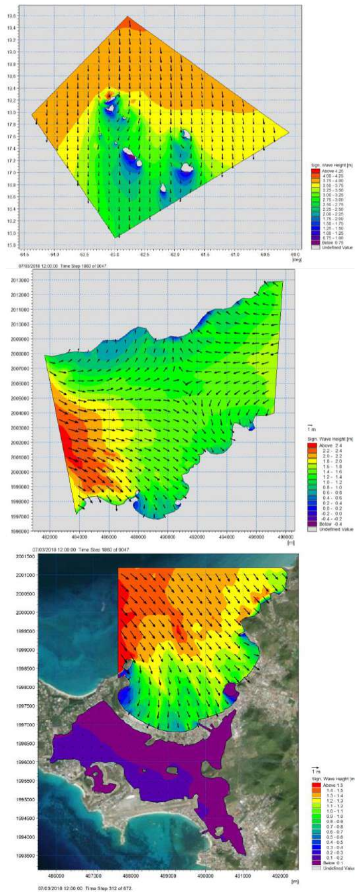
Figure 2.4 Chaîne de modélisation mise en œuvre : modèle régional (haut), modèle du Canal d'Anguilla (milieu), modèle de la baie de Galisbay (bas).
