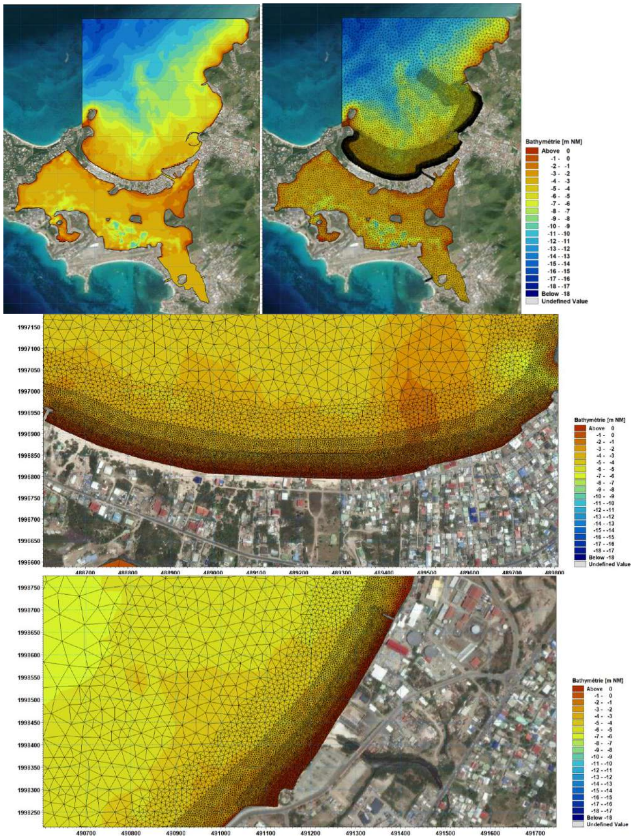
Figure 6.1 Emprise, bathymétrie interpolée et maillage du modèle hydrosédimentaire de la baie de Galisbay. Détails des plages de Sandy Ground et Galisbay.
