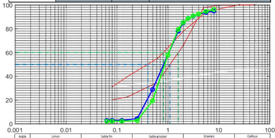
Figure 4.47 Courbes granulométriques des échantillons Ca8 – 0.5 m et Ca8 – 1.5 m (rouge), moyenne de la plage de Sandy Ground (bleu) et de la plage de Galisbay (vert).
