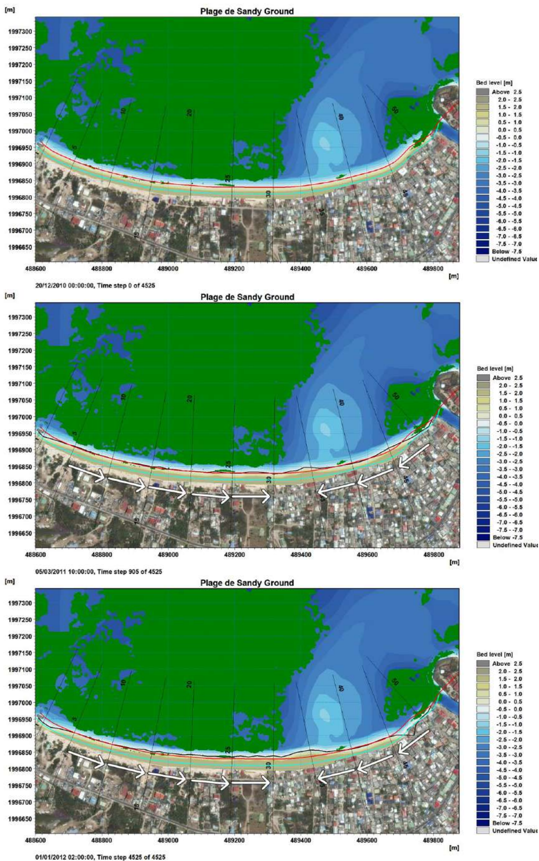
Figure 7.14 Évolution du rechargement de la plage de Sandy Ground : T0 (haut), après 1 an (milieu) et après 5 ans (bas).
