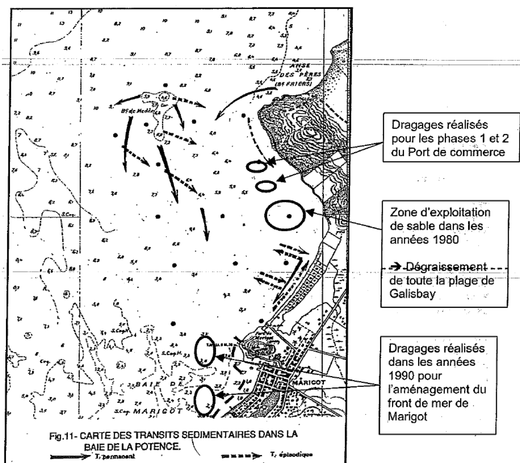
Figure 6.12 Carte des transits sédimentaires dans la Baie de la Potence (Réf. /4/).
