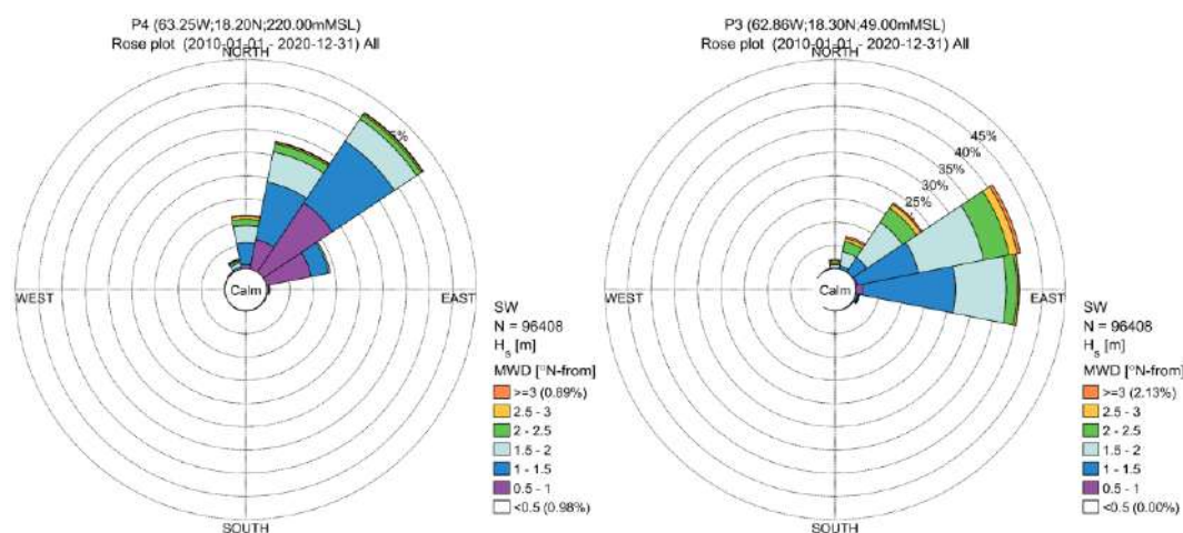
Figure 3.6 Roses des vagues modélisées aux points P4-NW (gauche) et P3-NE (droite) sur 2010-2020
