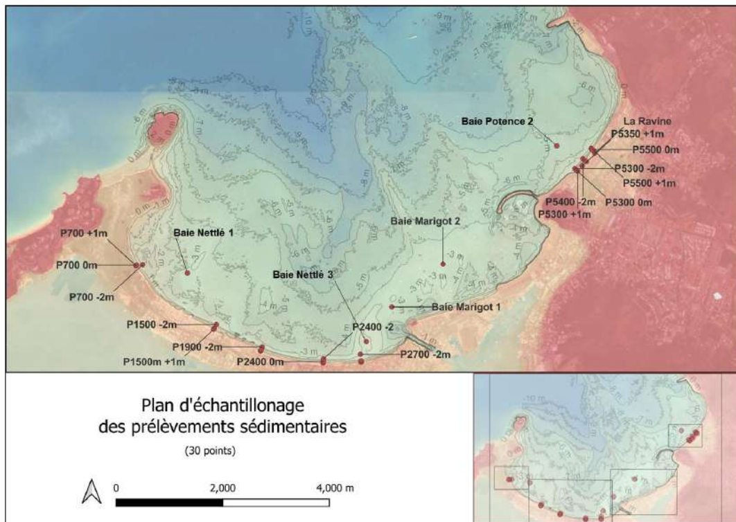
Figure 4.3 Carte des prélèvements sédimentaires
