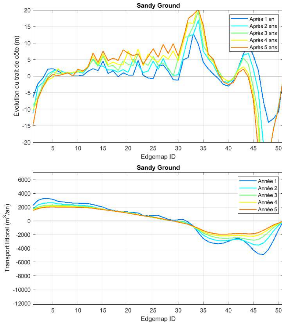
Figure 7.13 Evolution du trait de côte annuelle cumulée (haut) et dérive littorale annuelle (bas) sur la plage de Sandy Ground en 5 ans d'évolution morphodynamique après rechargement.
