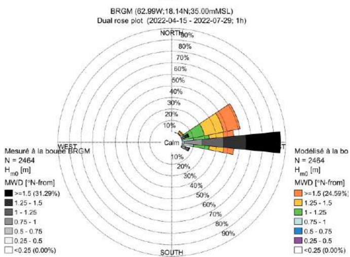
Figure 4.4 Roses des vagues mesurées (en grisé) et modélisées (en couleur) en B2 (ALIZE) et BRGM (Réf. /2/).
