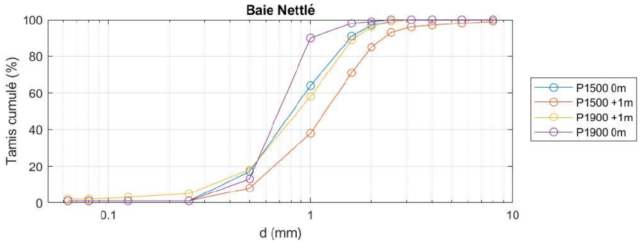
Figure 4.26 Courbes granulométriques des échantillons des plages de Baie Nettlé
