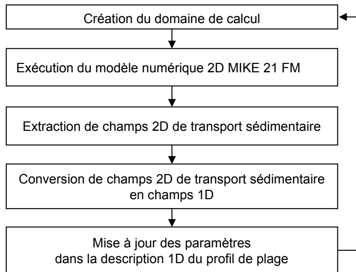
Figure 2.1 Cycle de fonctionnement du modèle hybride.
