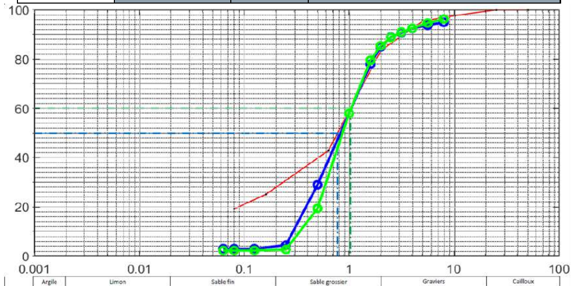
Figure 4.41 Courbe granulométrique de l'échantillon Ca2 – 0.5 m (rouge), moyenne de la plage de Sandy Ground (bleu) et de la plage de Galisbay (vert).
