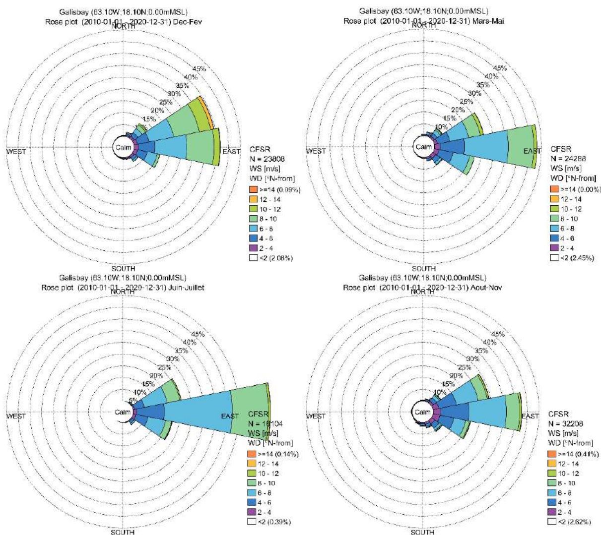
Figure 3.2 Roses des vents sur 2010-2020 à Saint-Martin, pour les quatre saisons – Données CFSR
