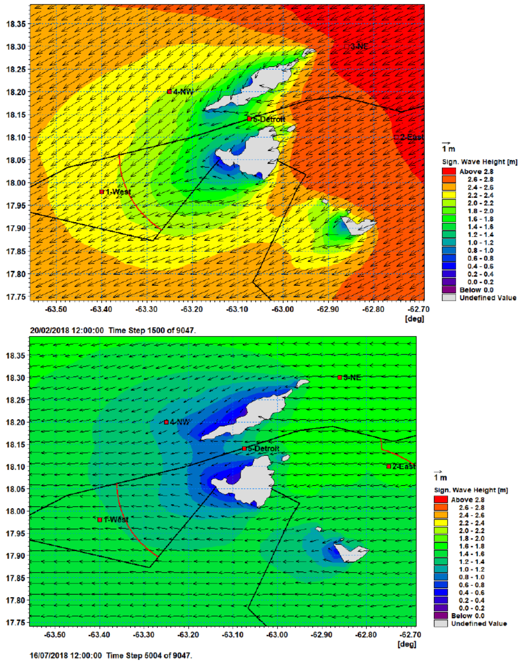
Figure 3.4 Champs de vagues du nord-est se réfractant autour de Saint-Martin et Anguilla : le 20/02/2018 lors d'Alizés de nord-est (en haut) et le 16/07/2018 en saison humide avec des vagues au large venant de l'est (en bas).
