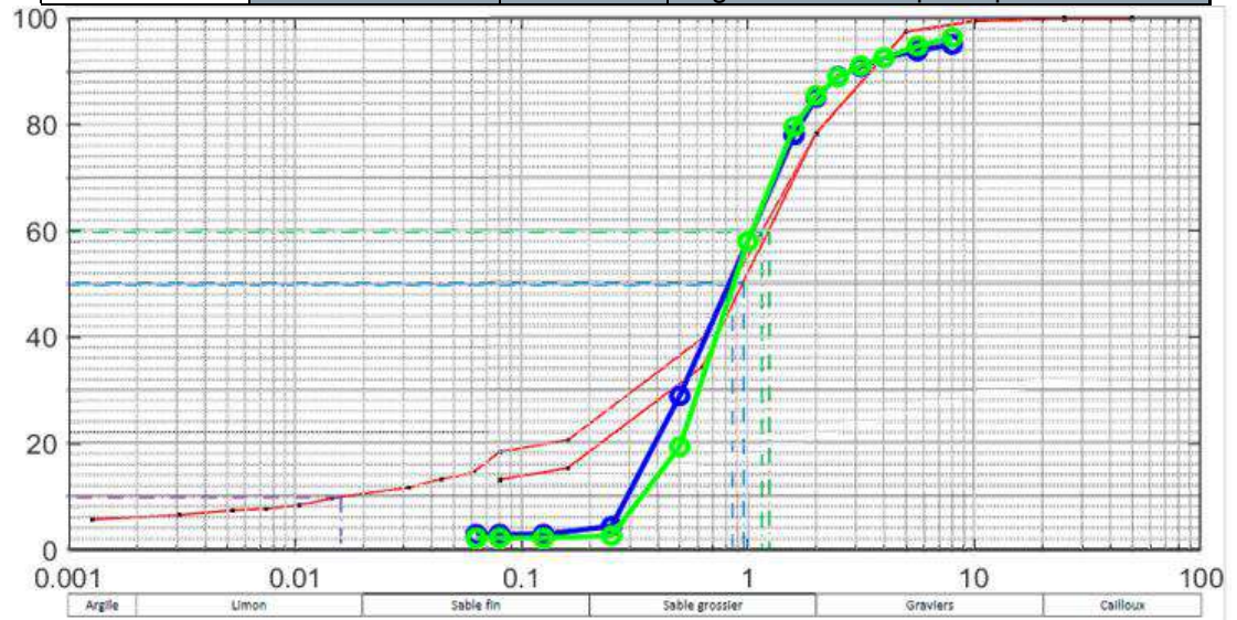
Figure 4.48 Courbes granulométriques des échantillons Ca1 – 1.6 m et Ca1 – 2.5 m (rouge), moyenne de la plage de Sandy Ground (bleu) et de la plage de Galisbay (vert).
