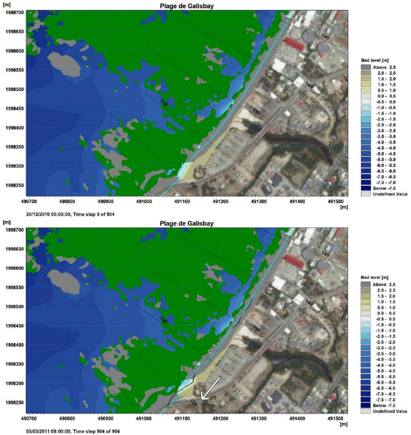
Figure 7.11 Plage de Galisbay à T0 (topo-bathymétrie Litto3D 2019) et après 1 an d'évolution morphodynamique
