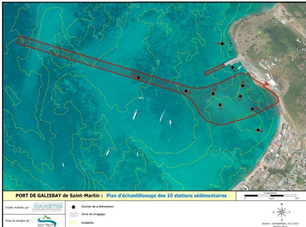
Figure 4.31 Plan d'échantillonnage des 10 stations de prélèvements (Réf. /19/).
