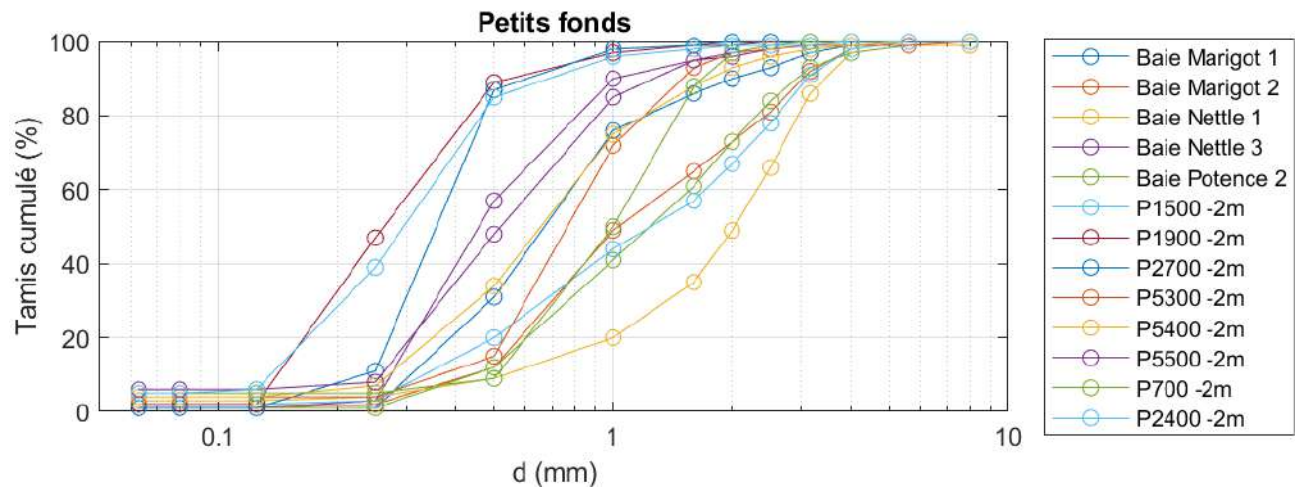
Figure 4.24 Courbes granulométriques des échantillons dans les petits fonds
