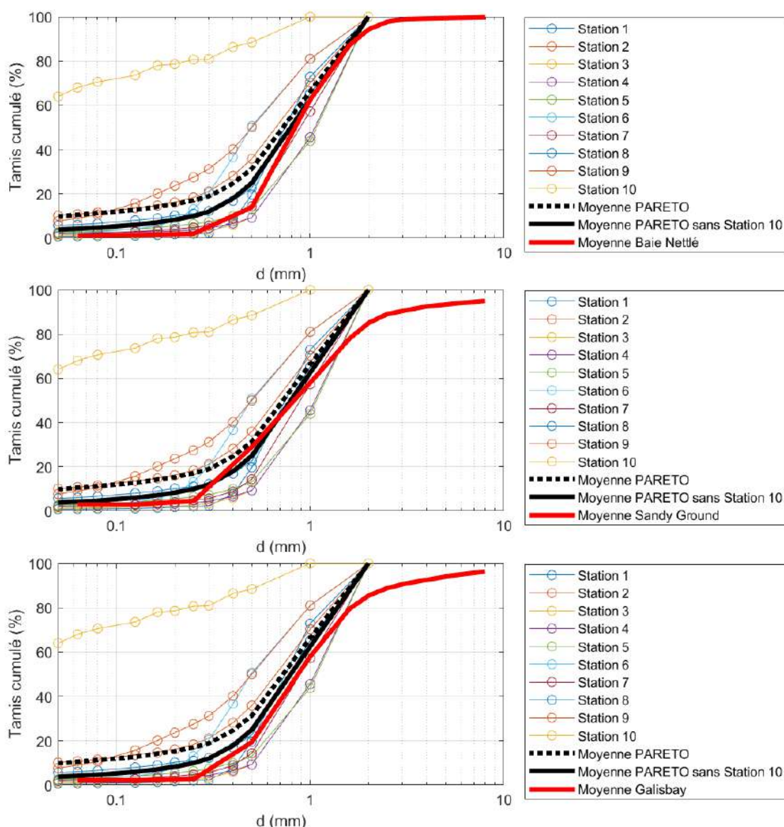
Figure 4.33 Comparaison entre les courbes granulométriques Pareto au site dragué et de la moyenne des courbes granulométriques Eurofins en Baie Nettlé (haut), Sandy Ground (milieu) et Galisbay (bas).
