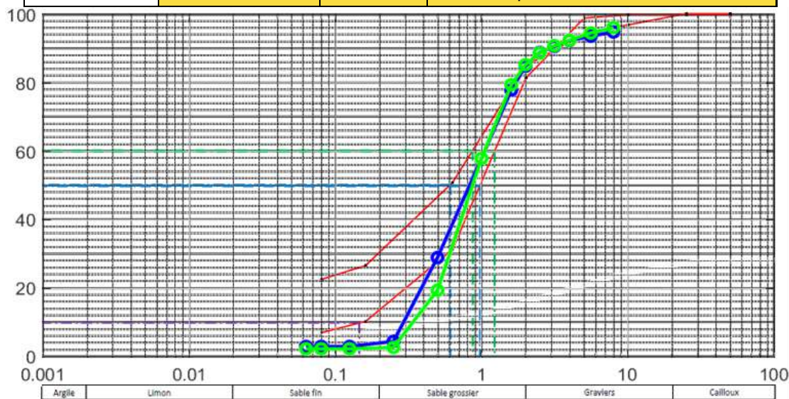
Figure 4.45 Courbes granulométriques des échantillons Ca6 – 0.5 m et Ca6 – 2.5 m (rouge), moyenne de la plage de Sandy Ground (bleu) et de la plage de Galisbay (vert).
