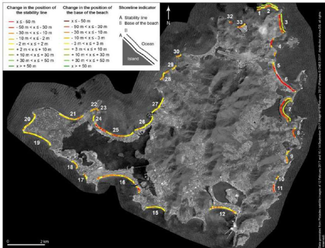
Figure 5.21 Impacts présumés des cyclones de septembre 2017 sur la position du trait de côte de l'île de Saint-Martin (Réf. /6/)
