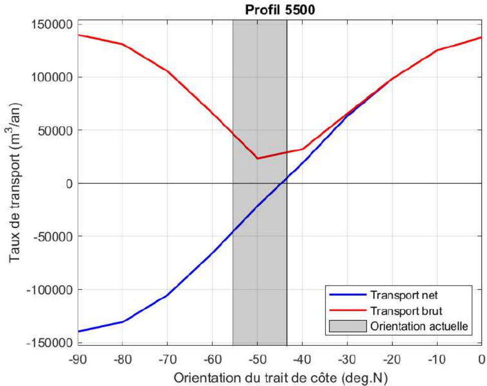
Figure 5.5 Transport net et brut annuel à travers le profil 5500 en fonction de l'orientation du trait de côte.
