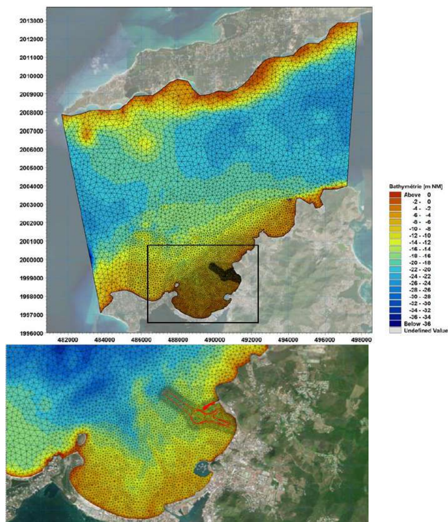
Figure 4.1 Emprise, bathymétrie interpolée et maillage du modèle hydrosédimentaire de la baie de Galisbay. Détails des plages de Sandy Ground et Galisbay.
