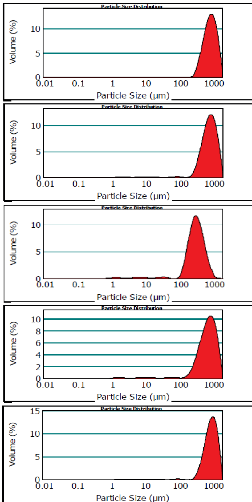
Figure 4.21 Courbes granulométriques obtenues par granulométrie laser. De haut en bas : P1500 0m, P2400 0m, P2400 -2m, P5300 0m, P5300 -2m.
