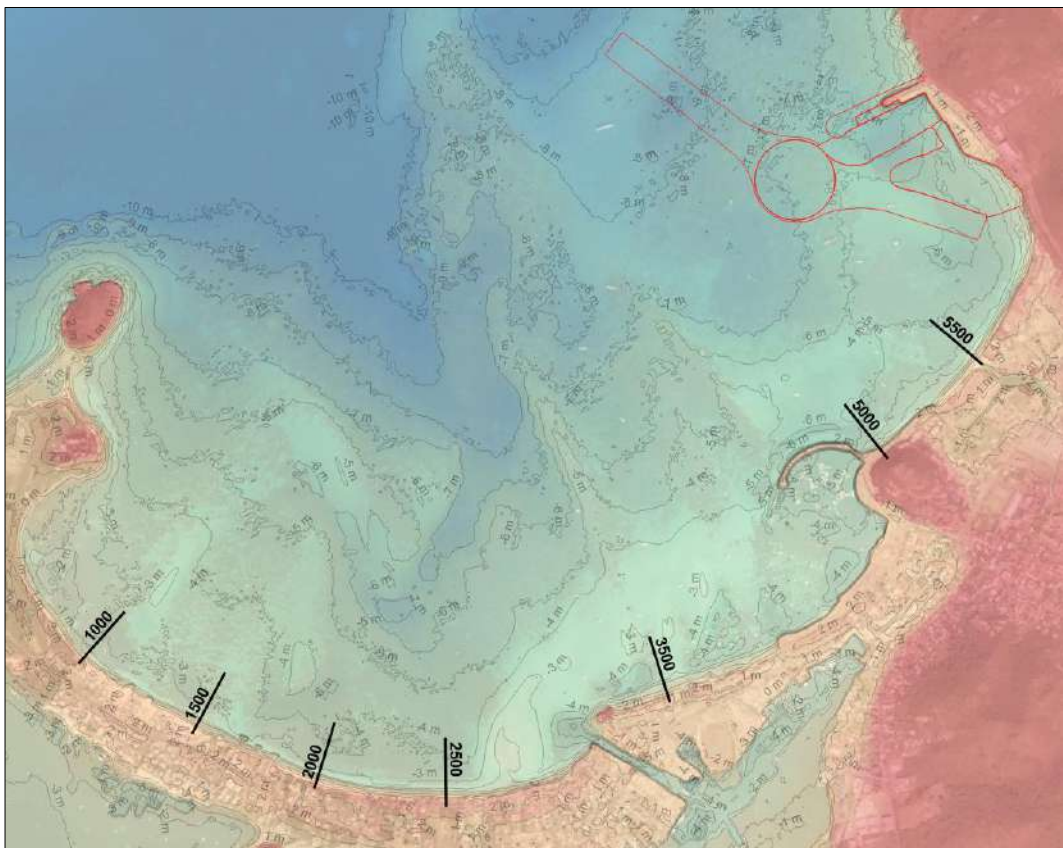
Figure 5.1 Emplacement des profils extraits pour la modélisation 1D du transport sédimentaire
