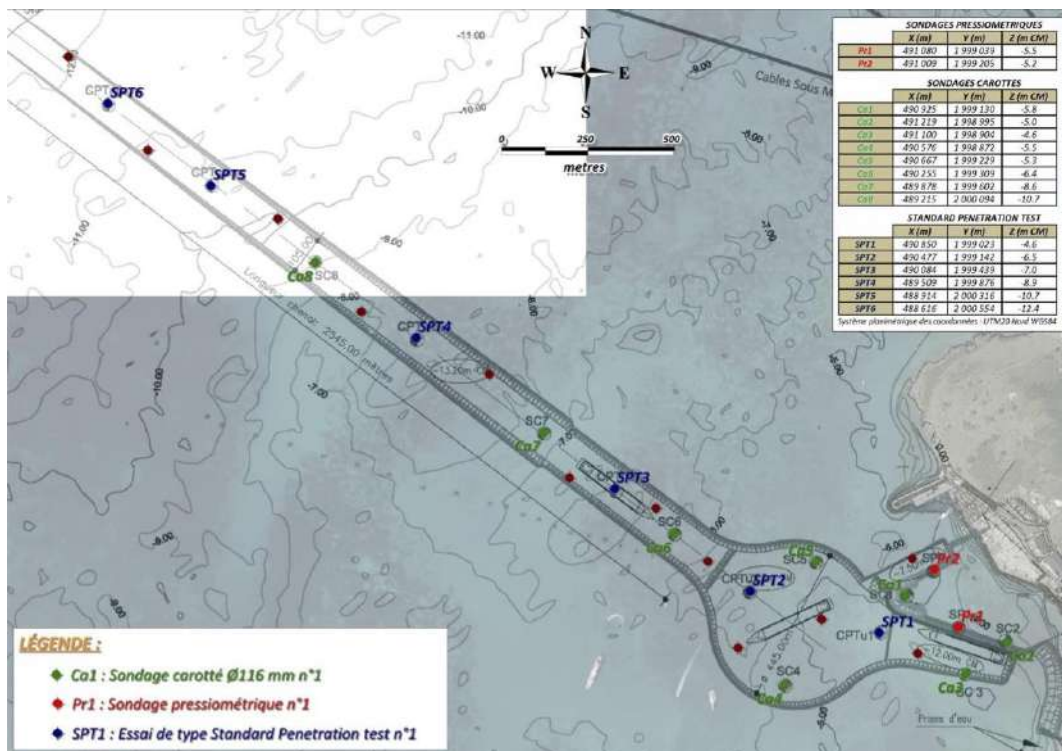
Figure 4.34 Plan d'implantation des reconnaissances géotechniques d'Antilles GEOTECHNIQUE 2016 (Réf. /1/)
