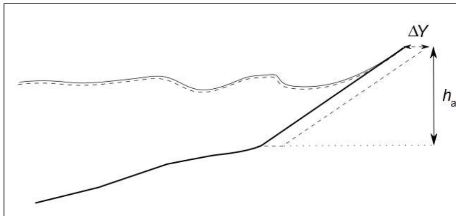
Figure 2.3 Illustration du principe de mise à jour de la position du profil côtier.
