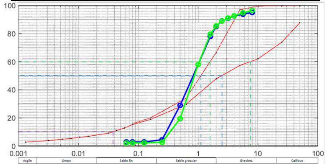
Figure 4.49 Courbes granulométriques des échantillons Ca2 – 0.5 m et Ca2 – 4 m (rouge), moyenne de la plage de Sandy Ground (bleu) et de la plage de Galisbay (vert).
