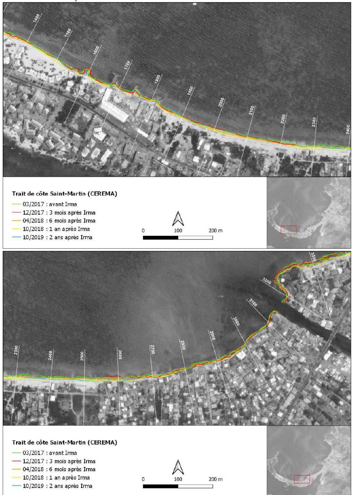
Figure 5.18 Traits de côte Cerema 2017-2019 Irma en Baie Nettlé et à Sandy Ground.
