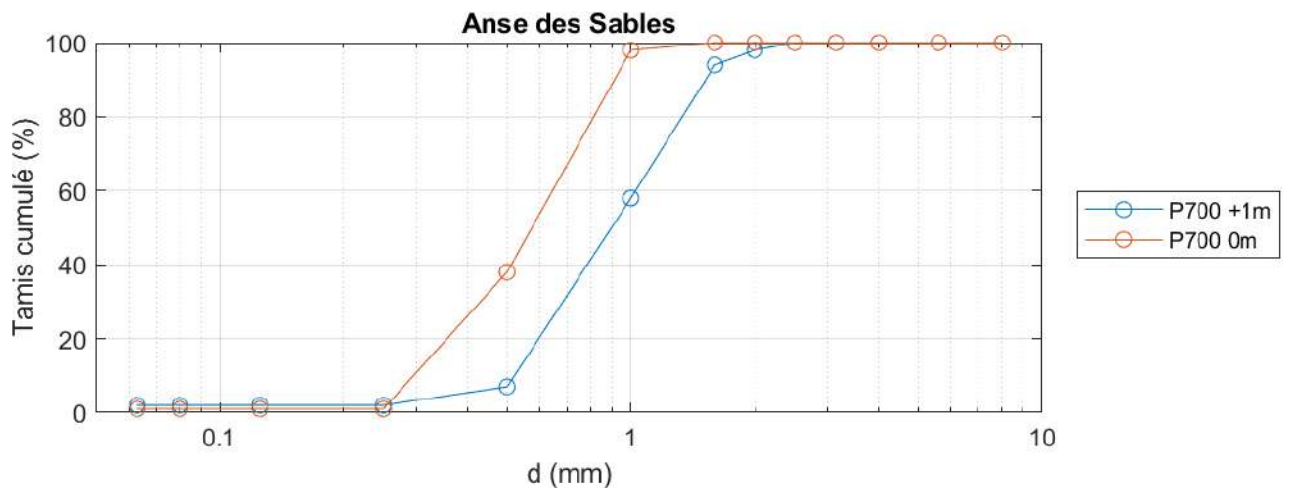
Figure 4.25 Courbes granulométriques des échantillons de la plage de l'Anse des Sables
