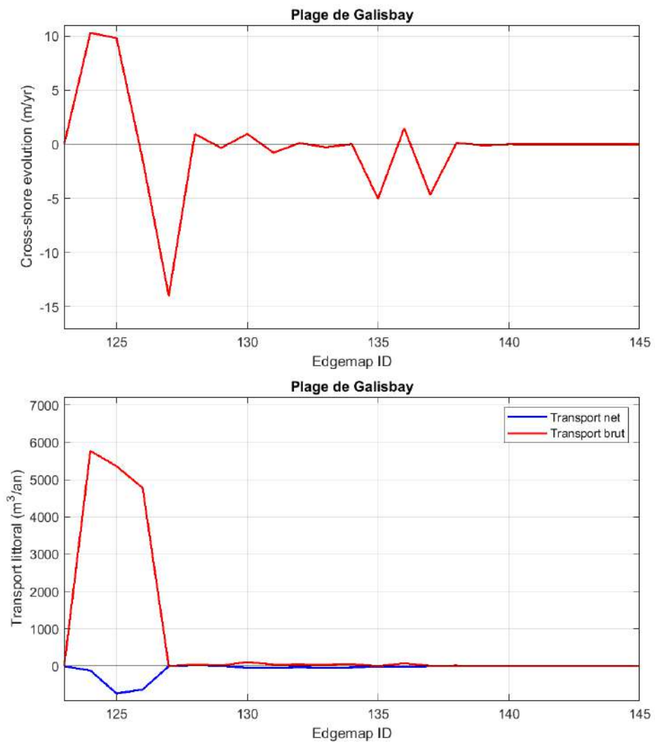
Figure 7.9 Evolution du trait de côte (haut) et dérive littorale (bas) sur la plage de Galisbay en 1 an d'évolution morphodynamique, état actuel.
