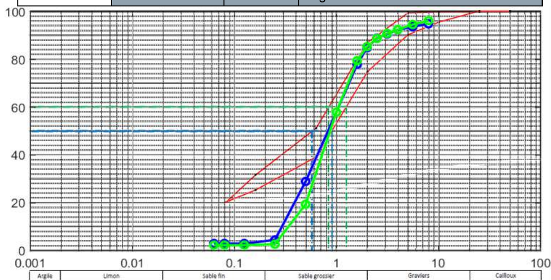
Figure 4.43 Courbes granulométriques des échantillons Ca4 – 0.5 m et Ca4 – 2.5 m (rouge), moyenne de la plage de Sandy Ground (bleu) et de la plage de Galisbay (vert).
