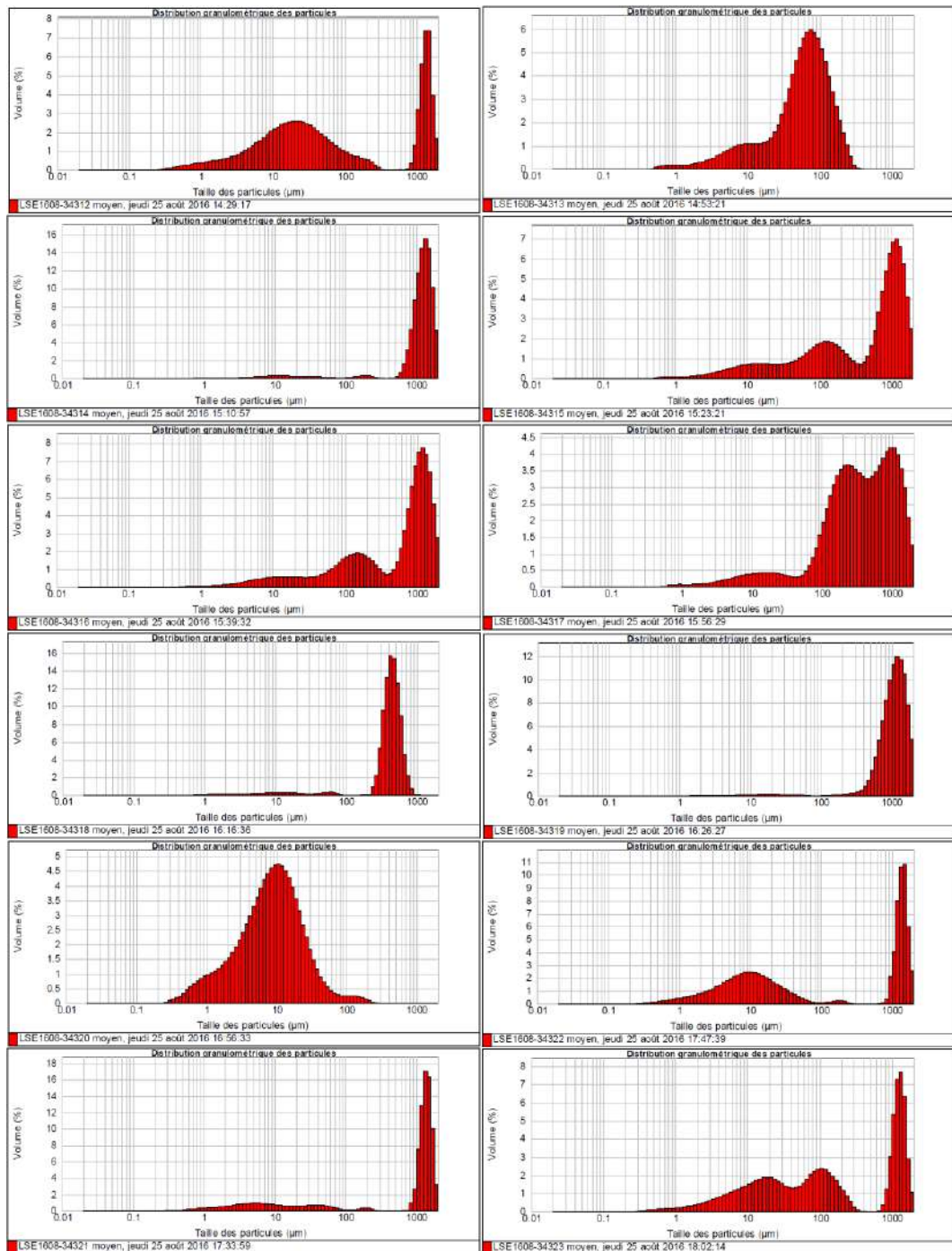
Figure 4.39 Distributions granulométriques dans la zone du projet à 0,5 m de profondeur (par plongeurs, Antilles-GEOTECHNIQUE, 2016), dans l'ordre de lecture : St1, St2, St3, St4, St5, St6, St7, St8, St9, St10, St11, St12 (Réf. /1/).
