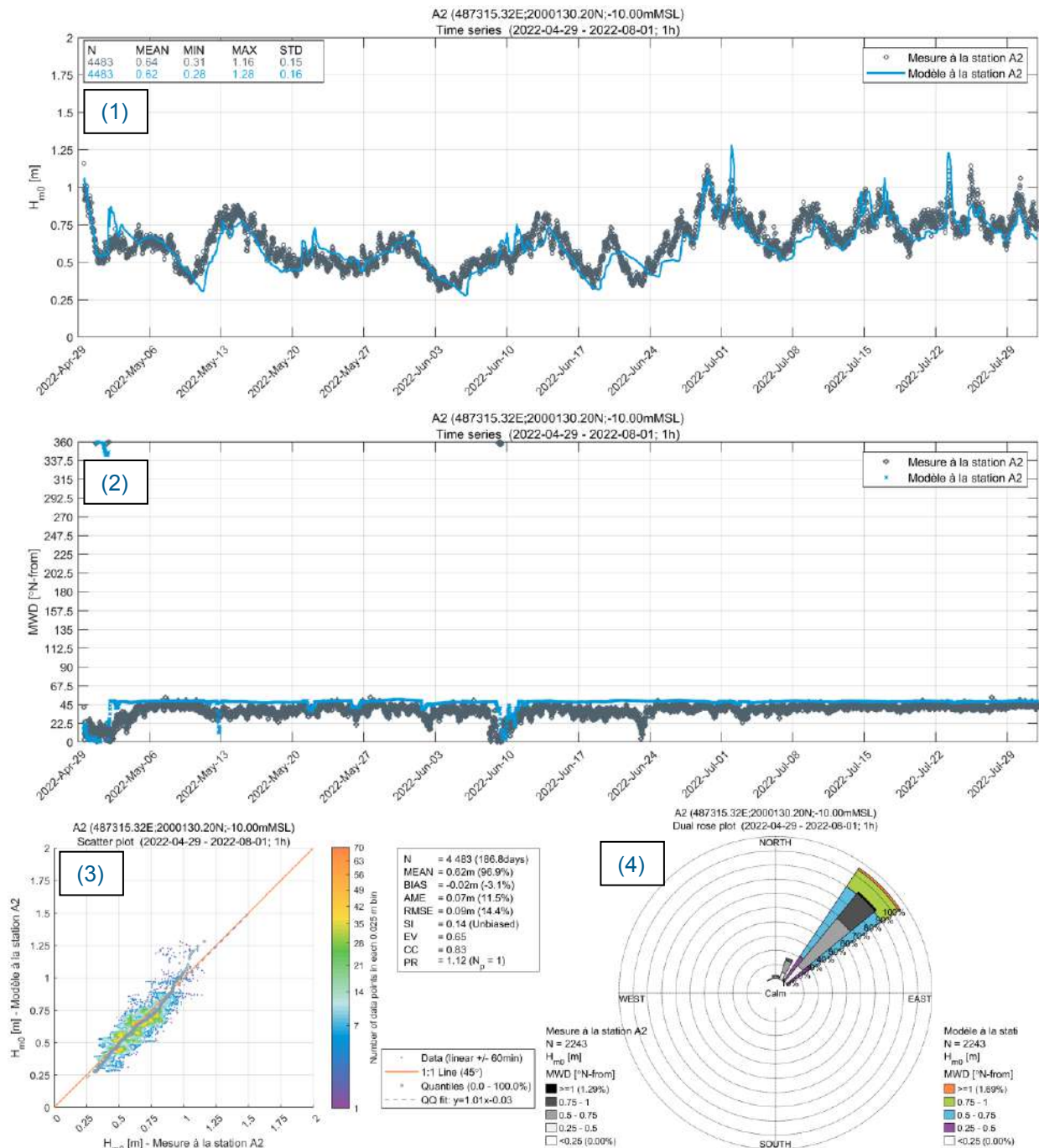
Figure 4.9 Comparaisons modèle-mesures en A2 sans décalage des directions de 14,7° : séries temporelles des hauteurs significatives (1) et des directions moyennes d'incidence (2) mesurées (en gris) et modélisées (en bleu), diagramme de dispersion des hauteurs significatives (3) mesurées versus modélisées, et roses des vagues (4) mesurées (en gris) et modélisées (en couleur).
