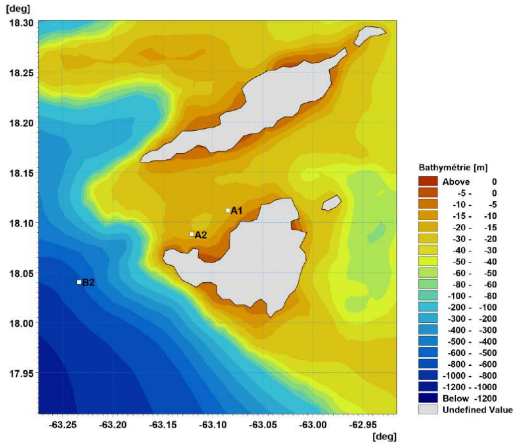
Figure 3.19 Position des stations de mesures de courants aux abords de Saint-Martin – campagne de mesures en cours.
