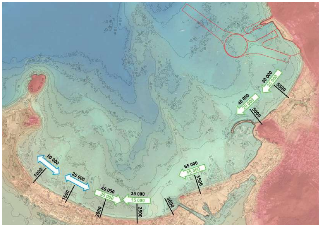
Figure 5.7 Schéma bilan du transport littoral brut le long du littoral de la baie de Galisbay. Les flèches indiquent le sens et l'intensité de la capacité de transport net annuel. Au-dessus des flèches est indiquée la capacité de transport brut annuel.
