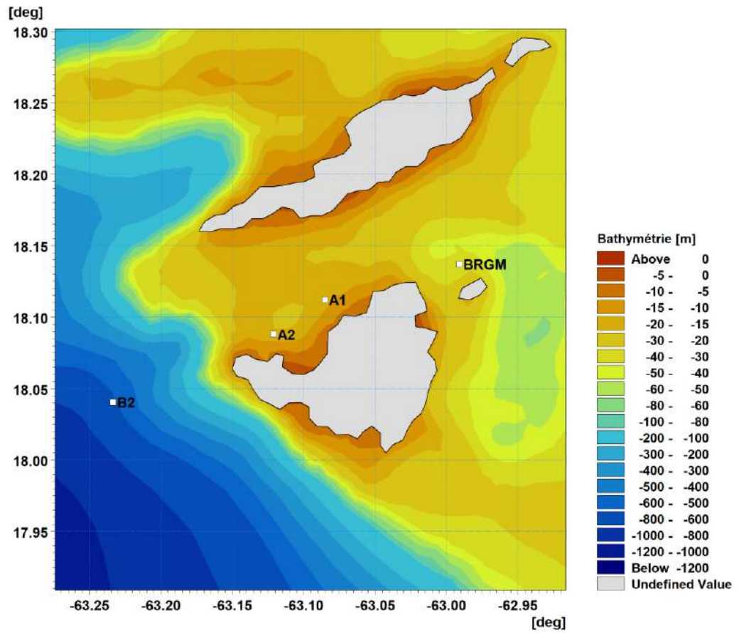
Figure 3.8 Position des stations de mesures de houle aux abords de Saint-Martin.
