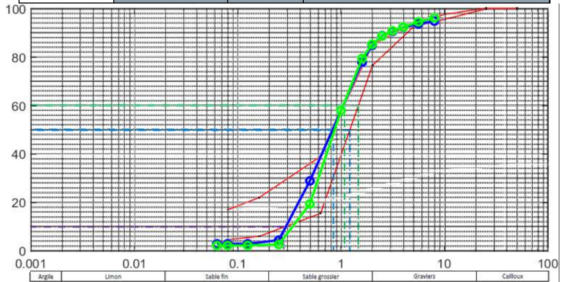
Figure 4.42 Courbes granulométriques des échantillons Ca3 – 0.5 m et Ca3 – 1.5 m (rouge), moyenne de la plage de Sandy Ground (bleu) et de la plage de Galisbay (vert).
