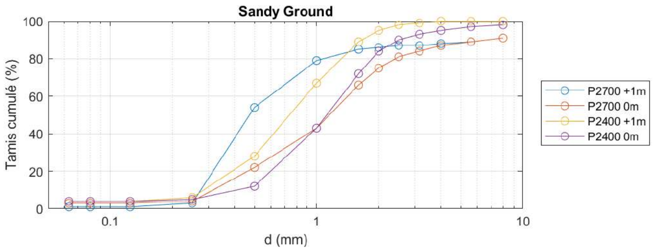
Figure 4.27 Courbes granulométriques des échantillons des plages de Sandy Ground
