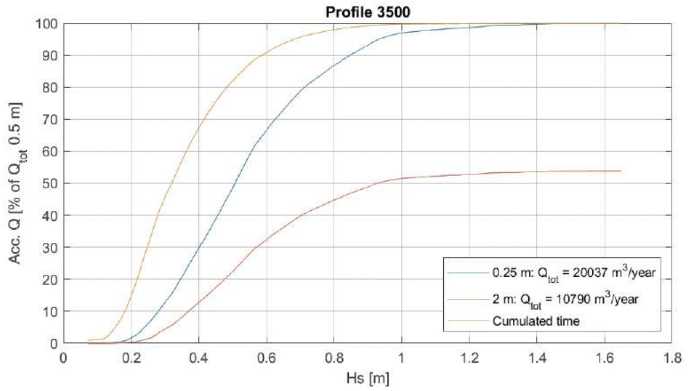
Figure 7.4 Transport brut cumulé à travers le profil 3500 pour une résolution de 0,25 m (bleu) et une résolution de 2 m (rouge) en pourcentage du transport brut total calculé pour la résolution la plus fine (0,25 m) et temps cumulé en pourcentage du temps total (jaune), en fonction de la hauteur de vague en pied de profil.
