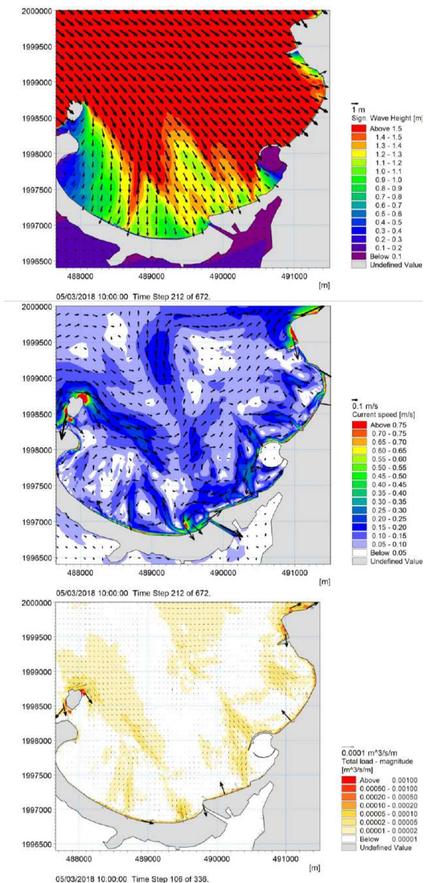
Figure 6.3 Champs de propagation des vagues (haut), des courants (milieu) et du transport sédimentaire (bas) le 05/03/2018 10h UTC lors d'un événement de Northers.
