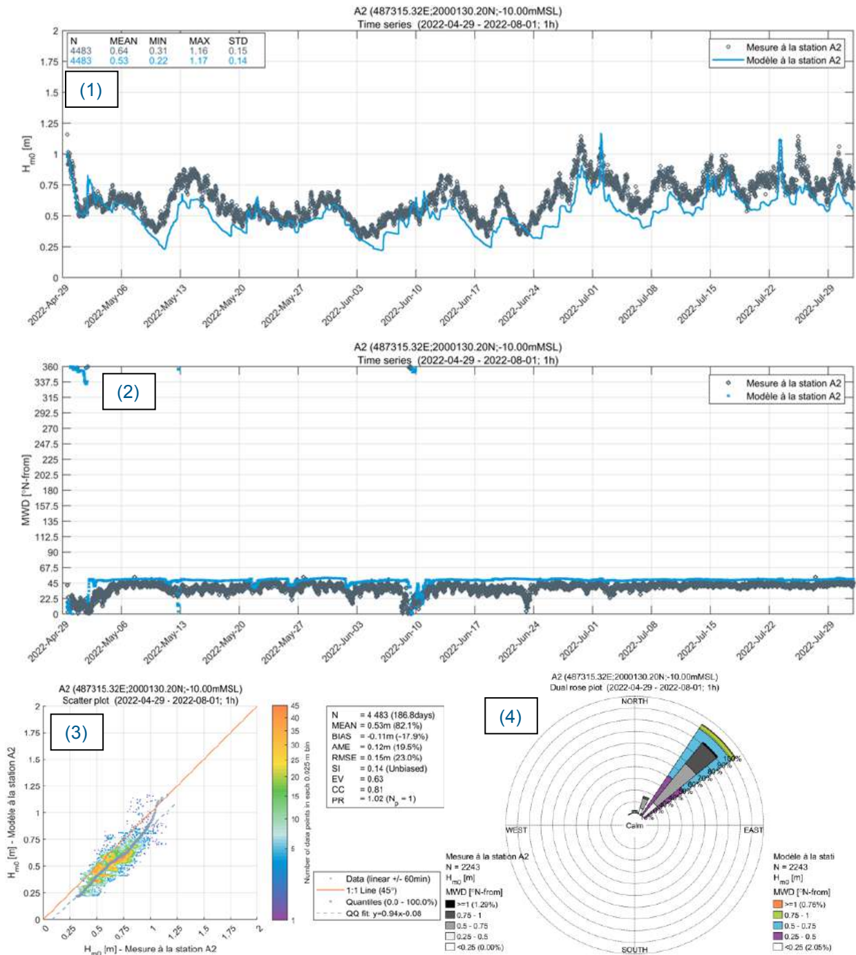
Figure 4.7 Comparisons modèle-mesures en A2 : séries temporelles des hauteurs significatives (1) et des directions moyennes d'incidence (2) mesurées (en gris) et modélisées (en bleu), diagramme de dispersion des hauteurs significatives (3) mesurées versus modélisées, et roses des vagues (4) mesurées (en gris) et modélisées (en couleur).
