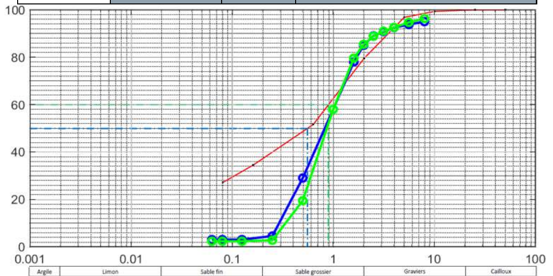
Figure 4.44 Courbe granulométrique de l'échantillon Ca5 – 0.5 m (rouge), moyenne de la plage de Sandy Ground (bleu) et de la plage de Galisbay (vert).
