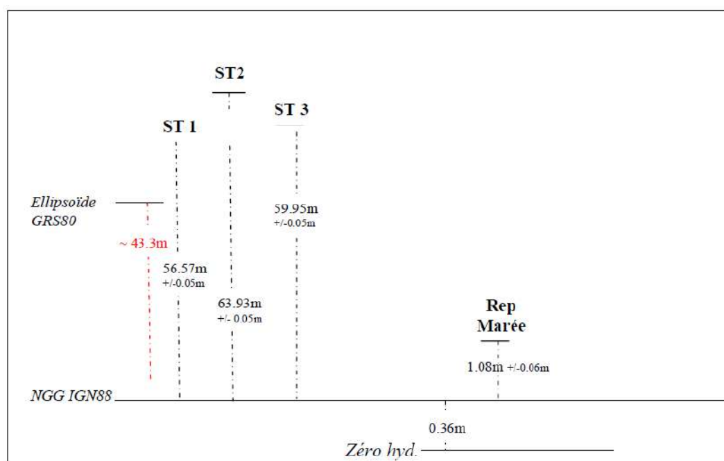
Figure 2.3 Schéma de rattachement des altitudes des repères géodésiques de Marigot (Réf. /14/)
