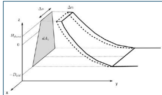
Figure 7.1 Schéma d'une section du trait de côte et définition des différents paramètres.
