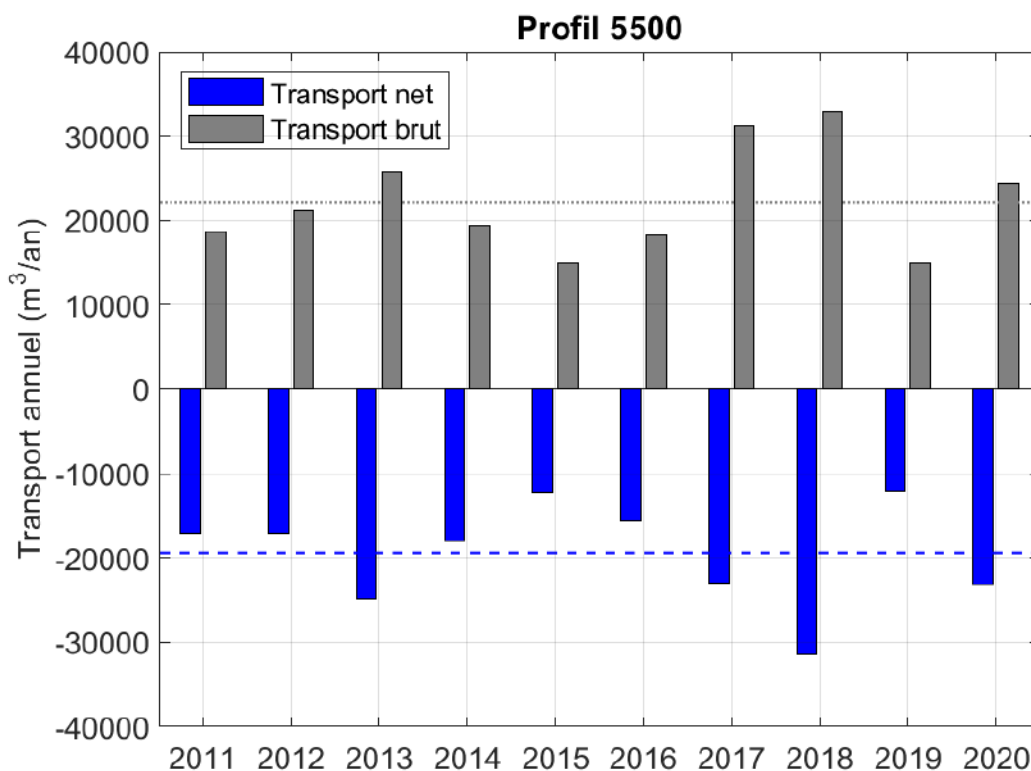
Figure 5.2 Variabilité interannuelle du transport sédimentaire net (en bleu, dirigé vers l'ouest lorsqu'il est négatif) et brut (en gris) sur la période 2011-2020 au profil 5500. Les lignes pointillées bleues et grises illustrent respectivement les transports net et brut moyens.
