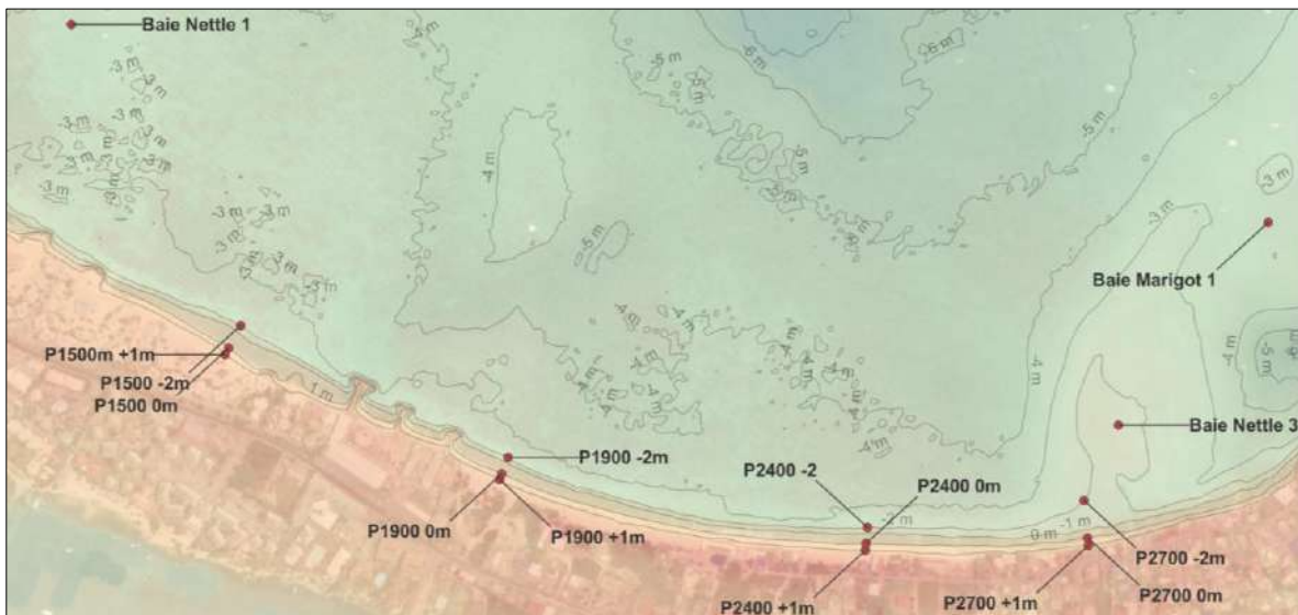
Figure 4.6 Position des prélèvements secteur Baie Nettlé
