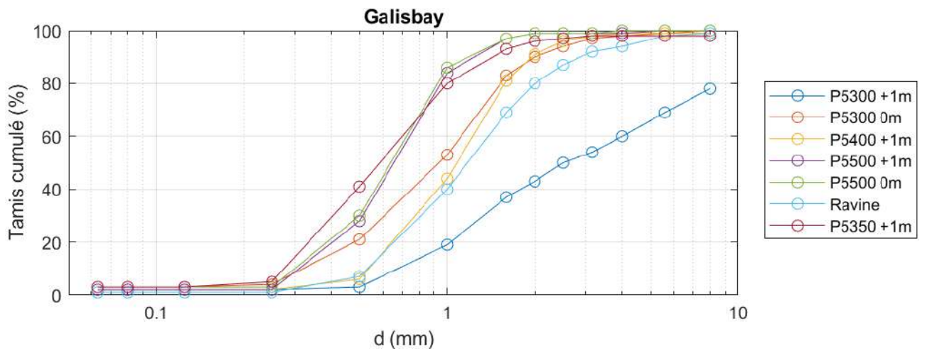
Figure 4.28 Courbes granulométriques de la plage de Galisbay
