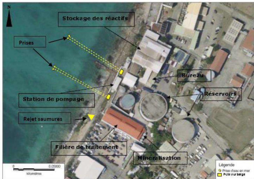
Figure 6.13 Schéma de l'usine de dessalement d'eau de mer de Galisbay (Réf. /21/)
