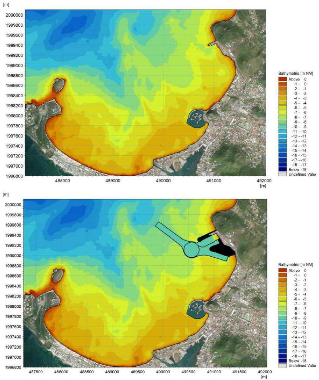
Figure 4.15 Configuration actuelle de la baie (haut) et configuration projet (bas).
