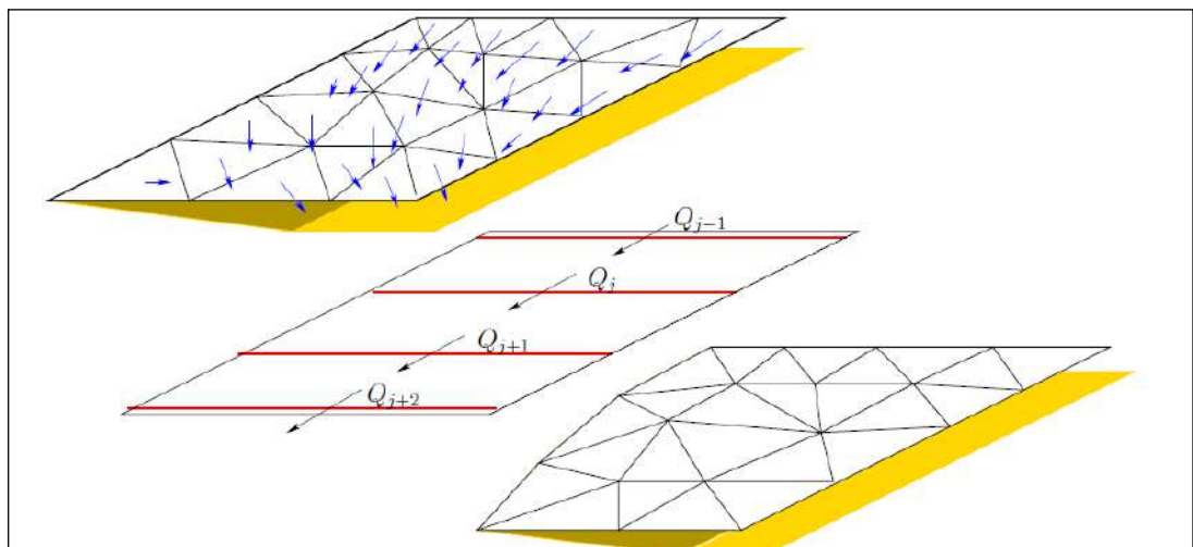
Figure 2.2 Illustration du principe de l'actualisation du maillage 2D dans l'approche hybride.
