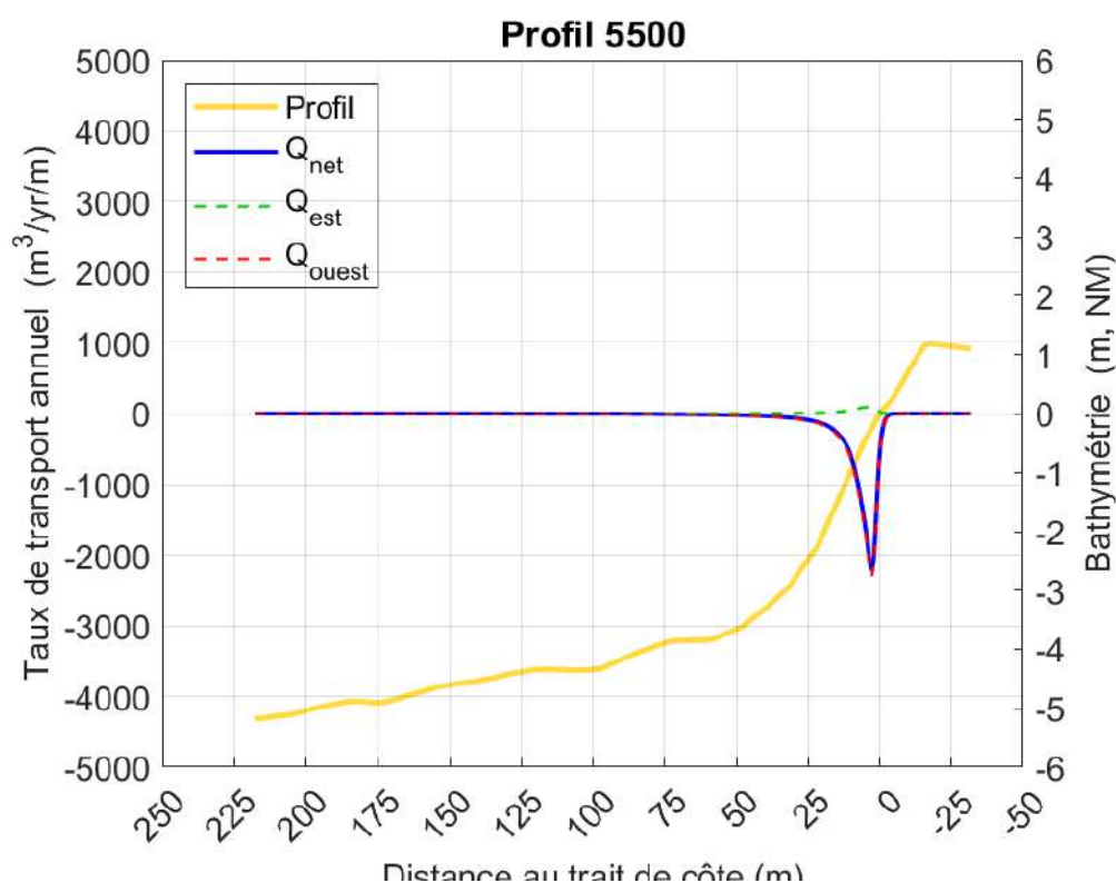
Figure 5.4 Distribution du transport sédimentaire dans le profil 5500 pour une orientation du trait de côte de 343 : transport vers l'est (vert), transport vers l'ouest (rouge), transport net (bleu).
