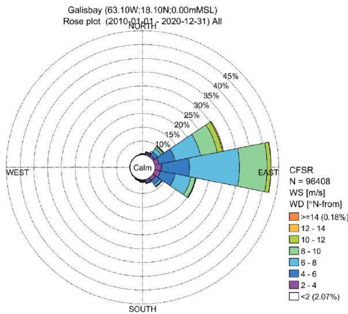
Figure 4.2 Rose des vents CFS 2010-2020 à Saint-Martin.
