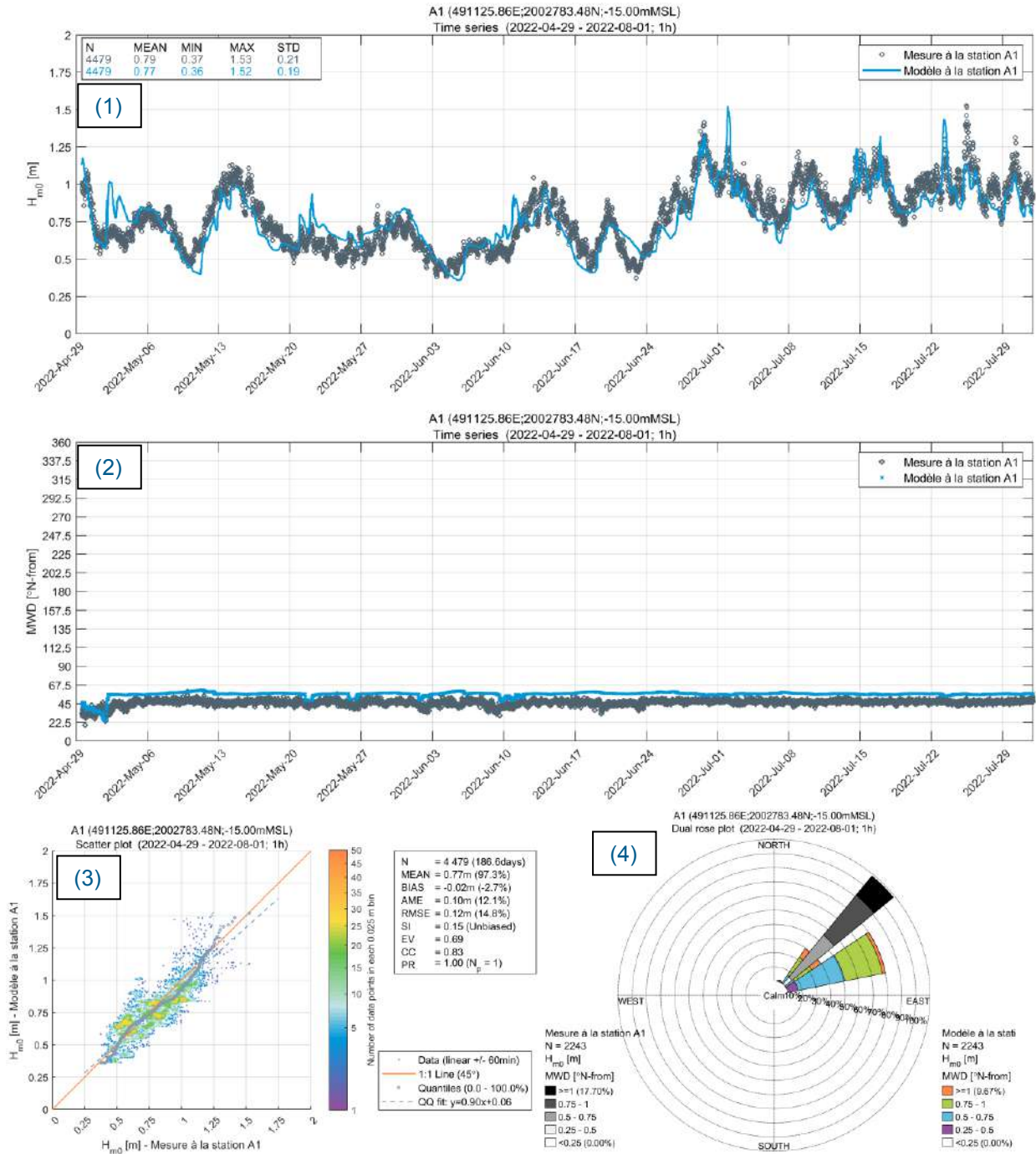
Figure 4.8 Comparisons modèle-mesures en A1 sans décalage des directions de 14,7 : séries temporelles des hauteurs significatives (1) et des directions moyennes d'incidence (2) mesurées (en gris) et modélisées (en bleu), diagramme de dispersion des hauteurs significatives (3) mesurées versus modélisées, et roses des vagues (4) mesurées (en gris) et modélisées (en couleur).
