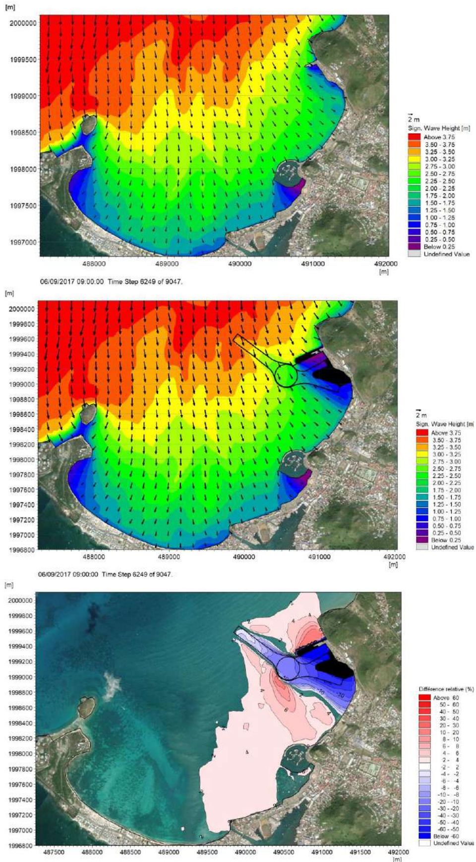
Figure 4.17 Champ de propagation des vagues le 06/09/2017 à 9h UTC pendant la tempête Irma en configuration actuelle de la baie (haut), configuration projet (milieu), et différence relative en pourcentage (bas).
