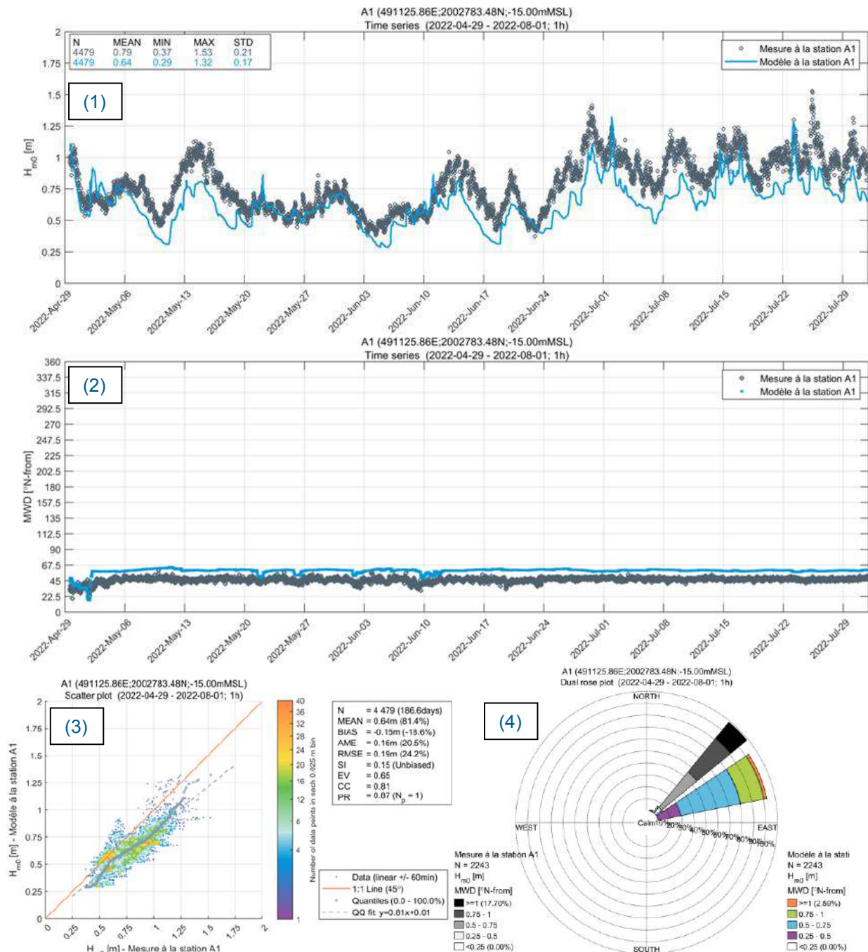
Figure 4.6 Comparisons modèle-mesures en A1 : séries temporelles des hauteurs significatives (1) et des directions moyennes d'incidence (2) mesurées (en gris) et modélisées (en bleu), diagramme de dispersion des hauteurs significatives (3) mesurées versus modélisées, et roses des vagues (4) mesurées (en gris) et modélisées (en couleur).
