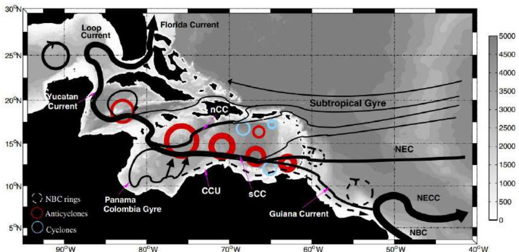
Figure 3.12 Illustration des principaux courants de la Mer des Caraïbes (NBC : Courant Nord Brésilien, NEC : Courant Nord Equatorial, nCC : Courant nord Caraïbe, SCC : Courant sud Caraïbe, CCU : Sous Courant Côtier) (Réf. /16/).
