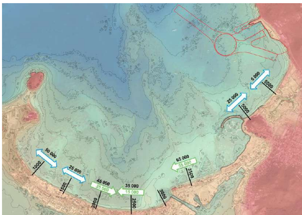
Figure 5.8 Schéma bilan du transport littoral brut le long du littoral de la baie de Galisbay en situation projet. Les flèches indiquent le sens et l'intensité de la capacité de transport net annuel. Au-dessus des flèches est indiquée la capacité de transport brut annuel.
