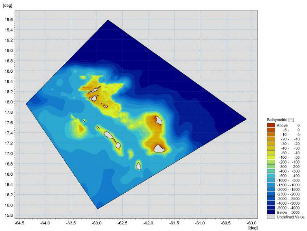
Figure 3.2 Bathymétrie interpolée du modèle régional de vagues de Saint-Martin.
