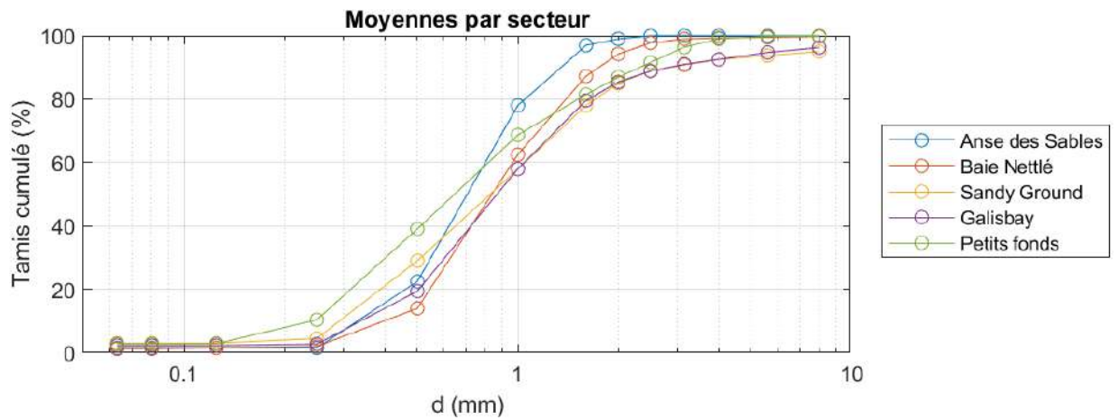
Figure 4.23 Courbes granulométriques moyennées par secteur.
