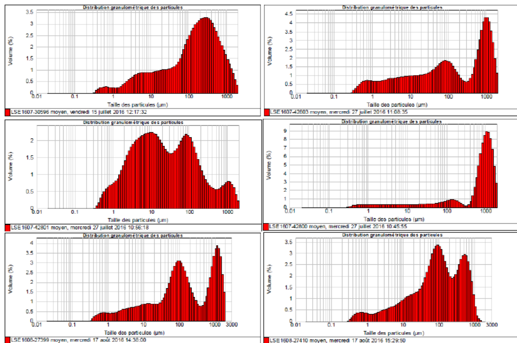
Figure 4.38 Distributions granulométriques dans la zone du projet (Antilles-GEOTECHNIQUE, 2016) dans l'ordre de lecture : Ca1-1,0 m, Ca4-3,5 m, Ca5-3,0 m, Ca6-2,7 m, Ca7-2,5 m, Ca8-3,0 m (Réf. /1/).
