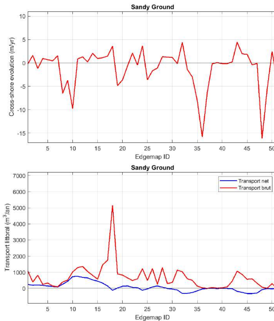
Figure 7.8 Evolution du trait de côte (haut) et dérive littorale (bas) sur la plage de Sandy Ground en 1 an d'évolution morphodynamique, état actuel.
