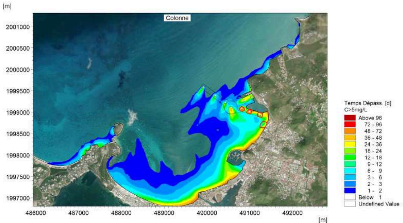
Figure 10 : Résultat de la simulation durant les 11,5 mois des travaux pour le calcul du temps de dépassement de la concentration de 5 mg/L de MES dans la colonne d'eau avec la mise en place de rideau anti-MES (source DHI)
