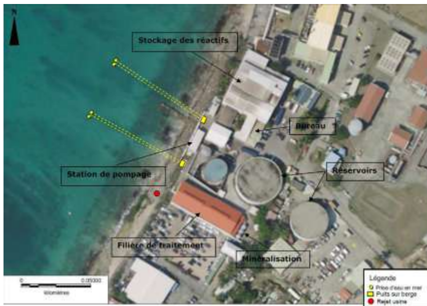
Figure 3 : Vue aérienne de l'usine. Seule une des deux conduites de pompage est opérationnelle (source Safège, 2014)
